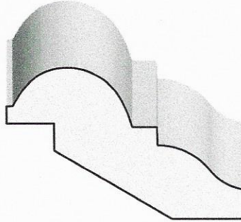
TS-PA 34 1 7/8 X 1 3/16
