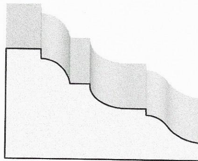
TS-CO 38 2 1/4 X 1 1/4
